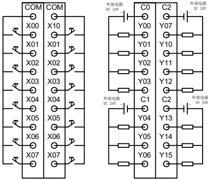
输入输出接线示意图
