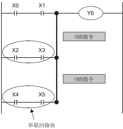
回路程序
