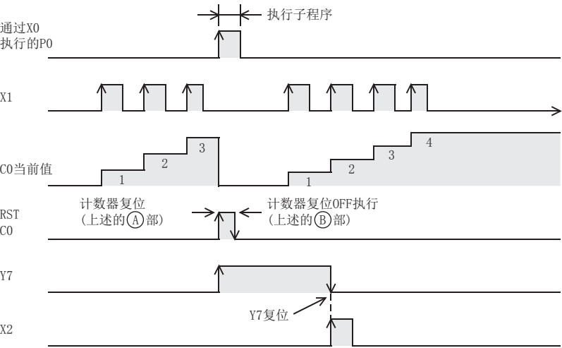
时序图
