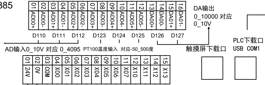
4.3寸一体机MC_20MR_6MT_FE430A_FX_F接线图
