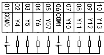
4.3寸一体机MC_20MR_6MT_FE430A_FX_F接线图
