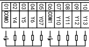
4.3寸一体机MC_20MR_6MT_F430A_FX_F接线图
