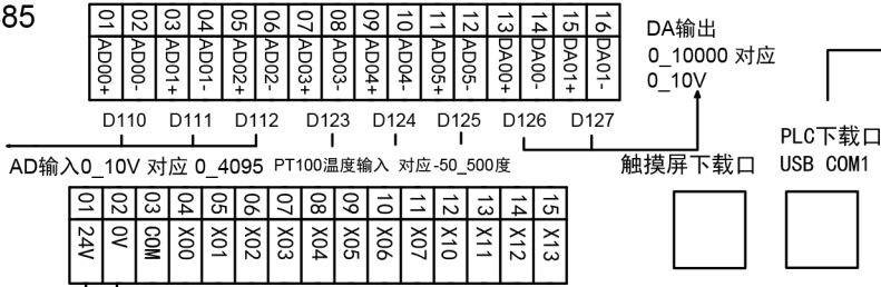
4.3寸一体机MC_20MR_6MT_F430A_FX_F接线图
