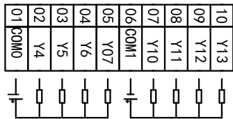
4.3寸一体机MC_20MR_6MT_F430A_FX3S_A接线图
