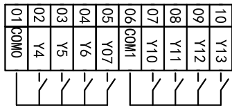
4.3寸一体机MM_20MR_6MT_430A_ES_B接线图
