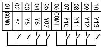
4.3寸一体机MM_20MR_6MT_430A_ES_A接线图
